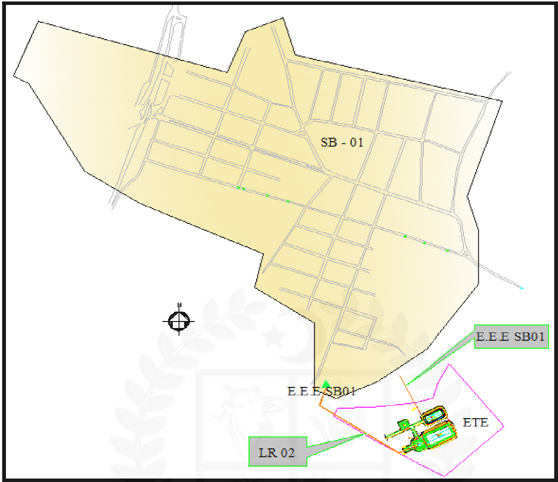
Figura 13.2 – Concepção do SES de Luzinópolis - 2017
