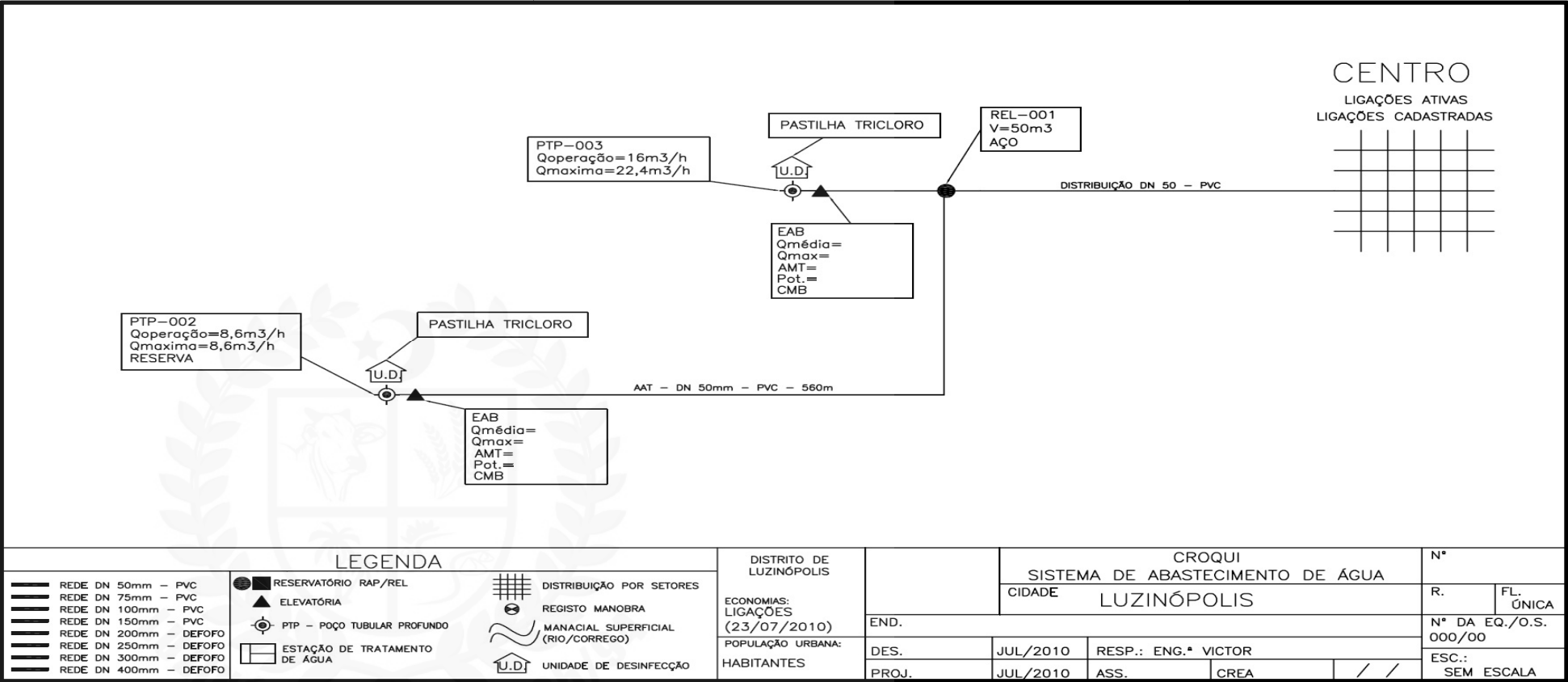
Figura 13.1 - Croqui do Sistema de Abastecimento de Água Existente
